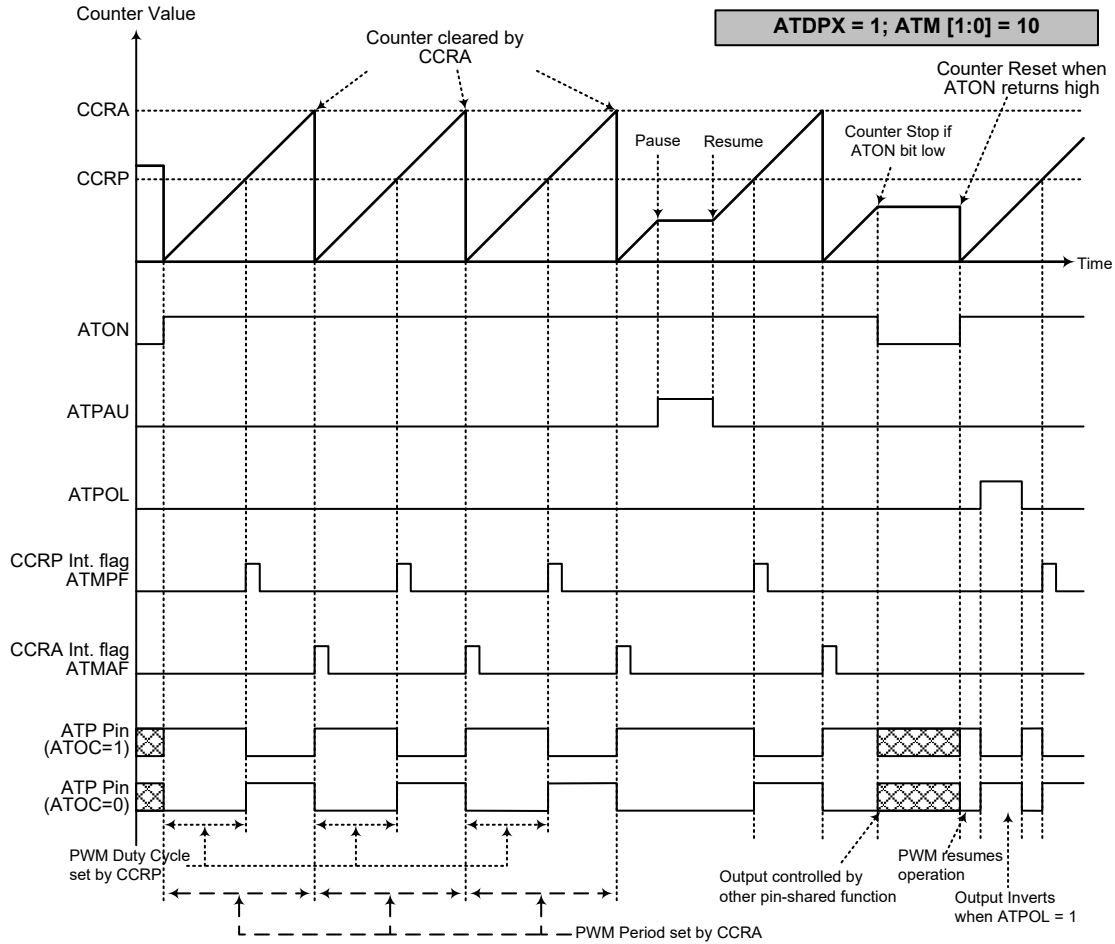
ATM 正常 PWM 输出模式 - ATDPX=1
