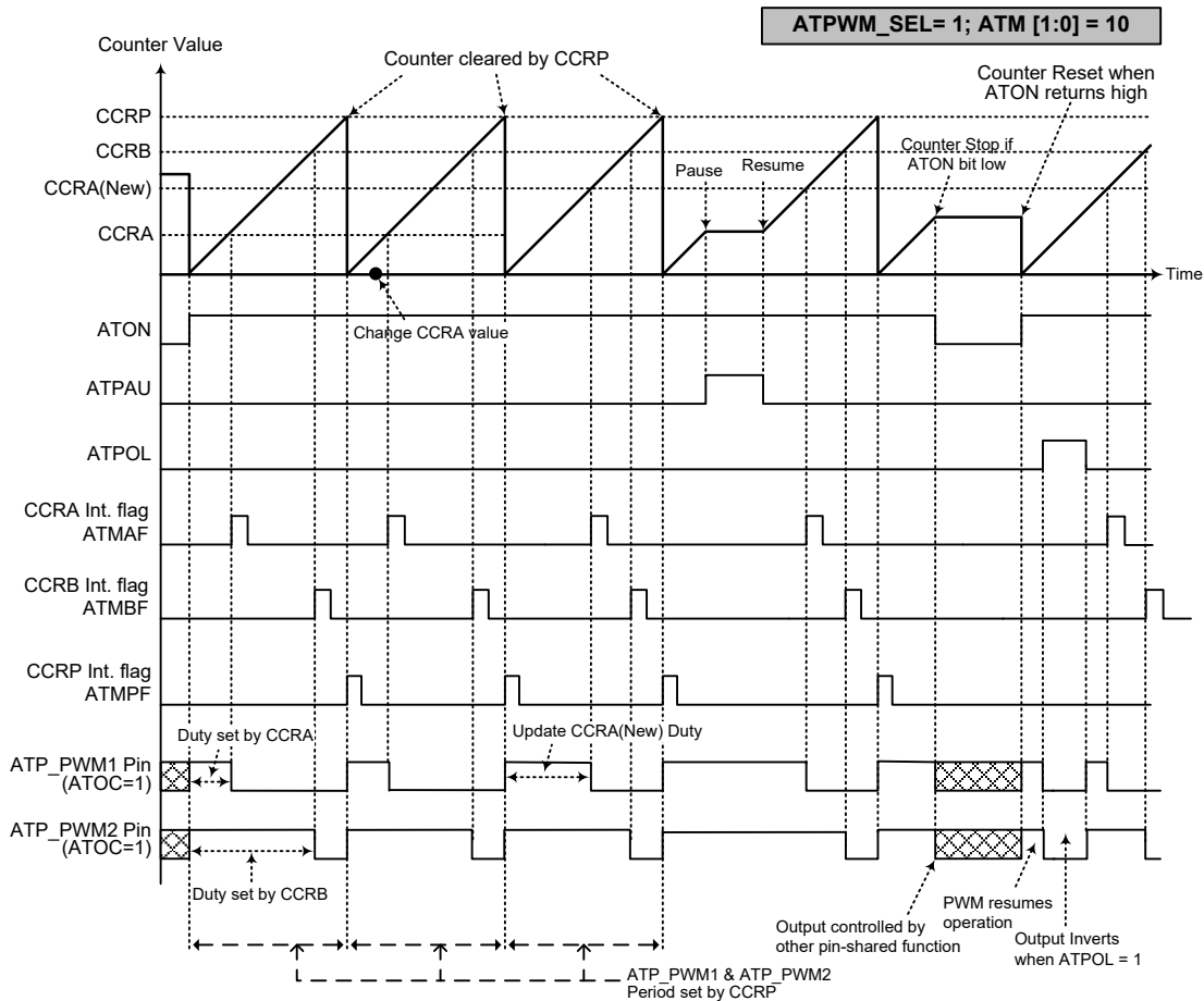
ATM 音频 PWM 输出模式 – 改变 CCRA 值
