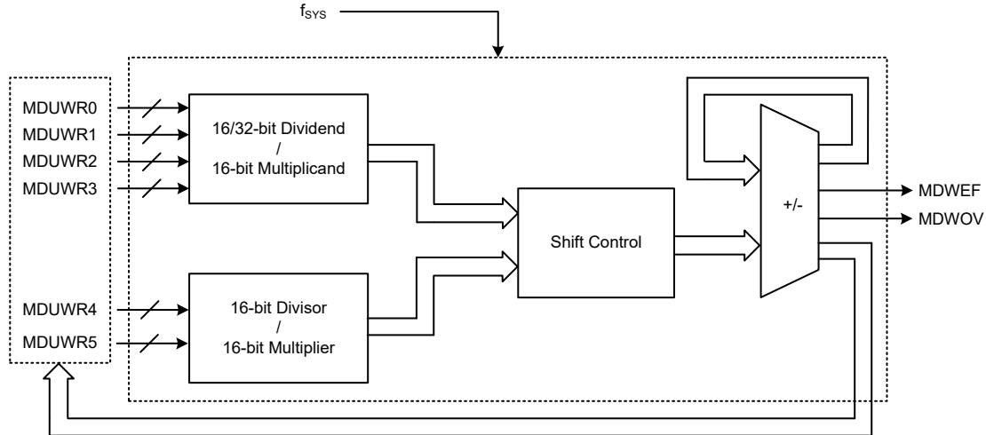
16-bit MDU 方框图
