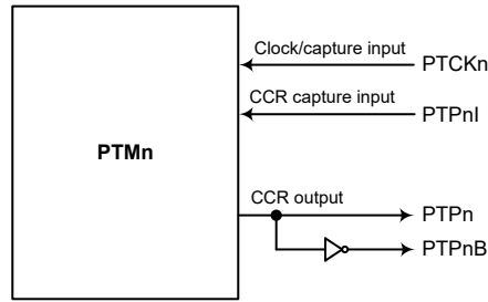
PTMn 功能引脚框方图 (n=0~2)
