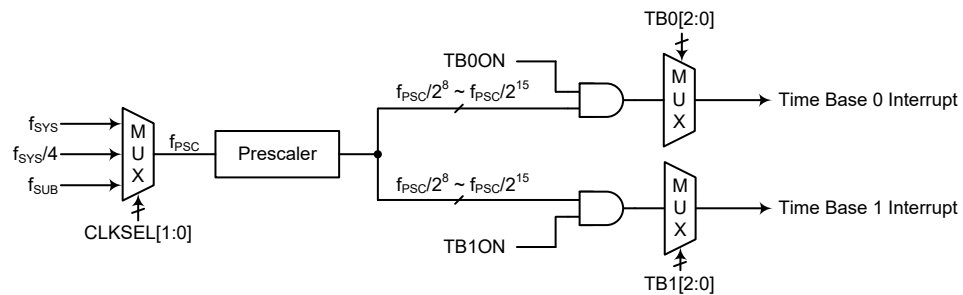
时基中断
