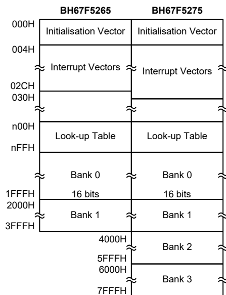
程序存储器结构
