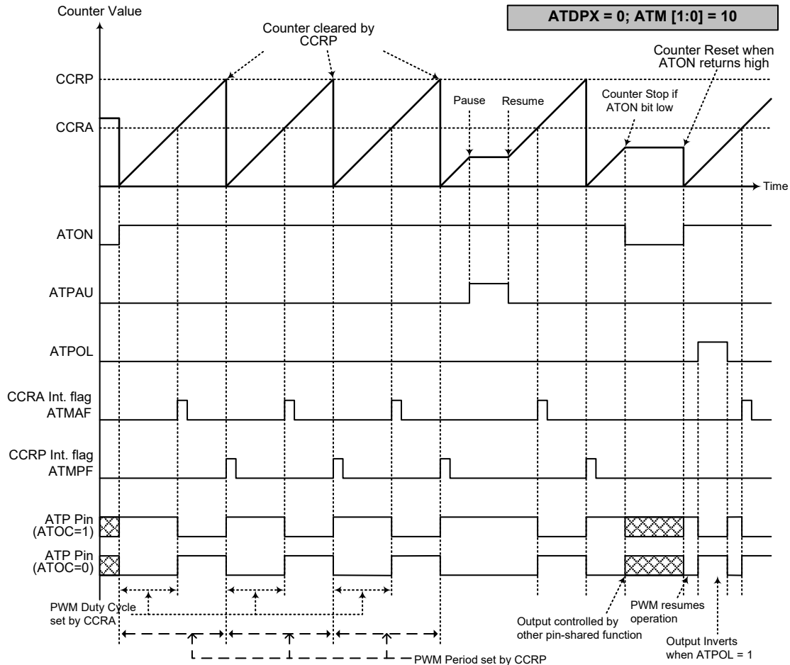
ATM 正常 PWM 输出模式 – ATDPX=0
