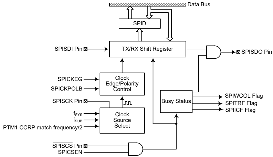
SPI 方框图
