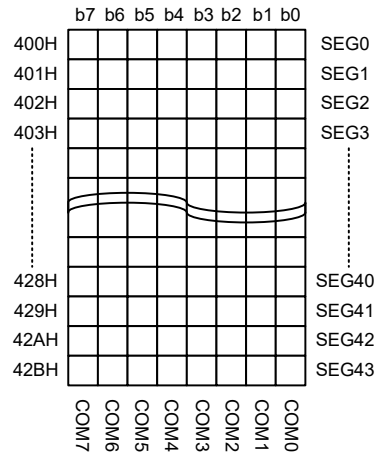
LCD 存储器映射图 - BH67F5275
