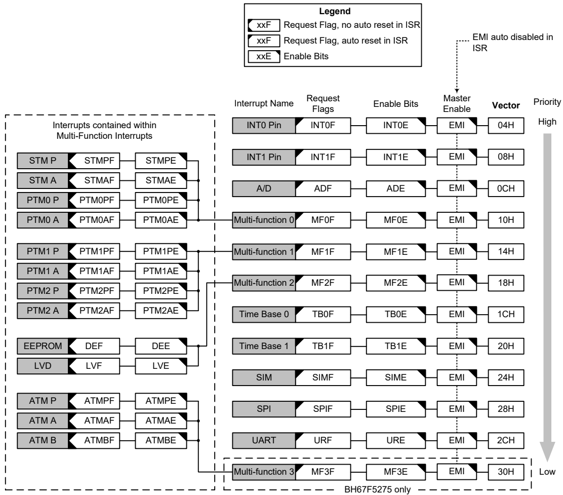
中断结构
