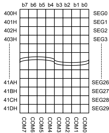
LCD 存储器映射图 - BH67F5265
