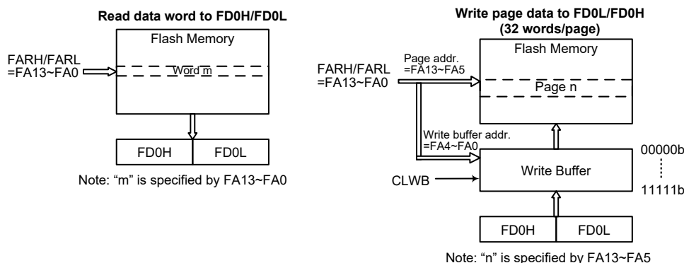
Flash 存储器 IAP 读 / 写结构 – BH67F5265
