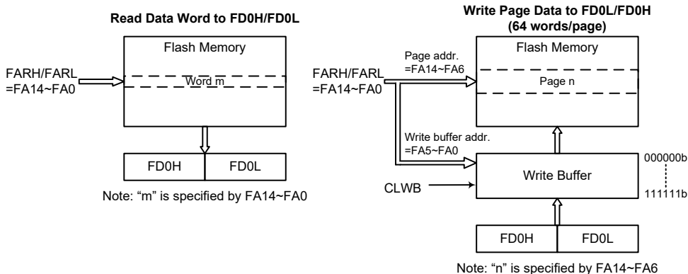
Flash 存储器 IAP 读 / 写结构 – BH67F5275
