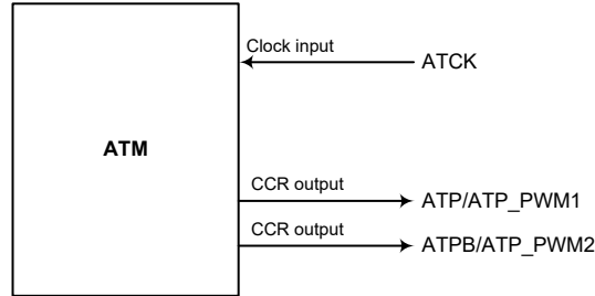
ATM 功能引脚方框图 - BH67F5275
